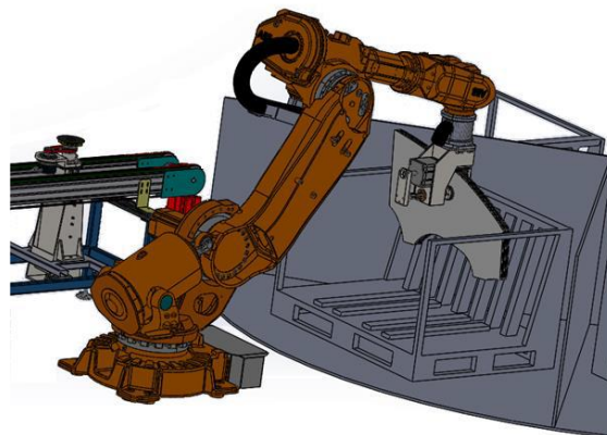
Automatizace balení kalených skel na lince bočních autoskel (D. Jaroš, 2020)
