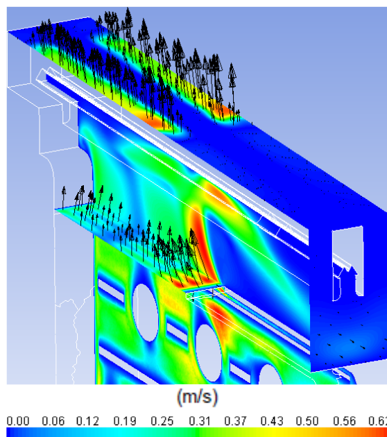
Analýza proudění vzduchu uvnitř podlahového konvektoru a v jeho okolí (J. Egert, 2015)
